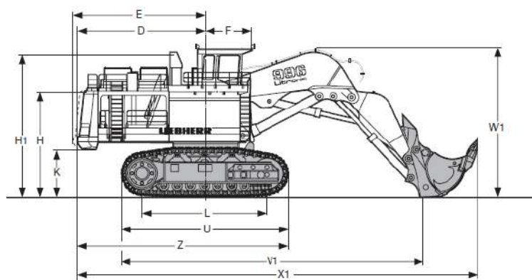
شکل ۱- بیل مکانیکی
