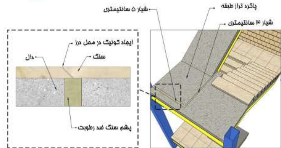
نمونه اجرای سنگ در پاکرد تراز طبقه در ممل درز
