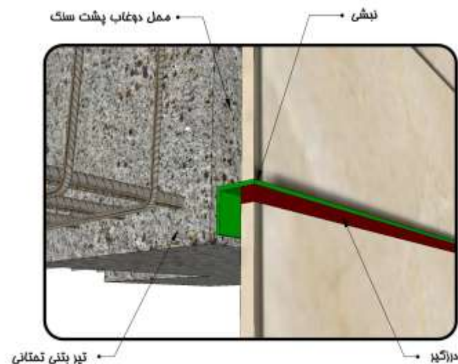
جزئیات اتصال نبشی نگهدارنده سنگ به تیر بتنی تمثالی
