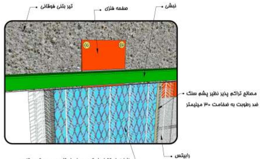
جزئیات استقرار رابیتس و پلی استایرن روی ستون بتنی
