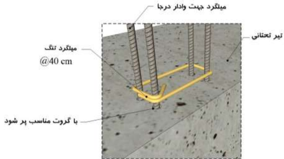
■ کاشت میلگرد روی تیر تحتانی (پیشنهاد دوم)
