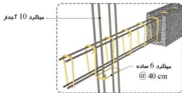
تقاطع وادر با نعل درگاه
