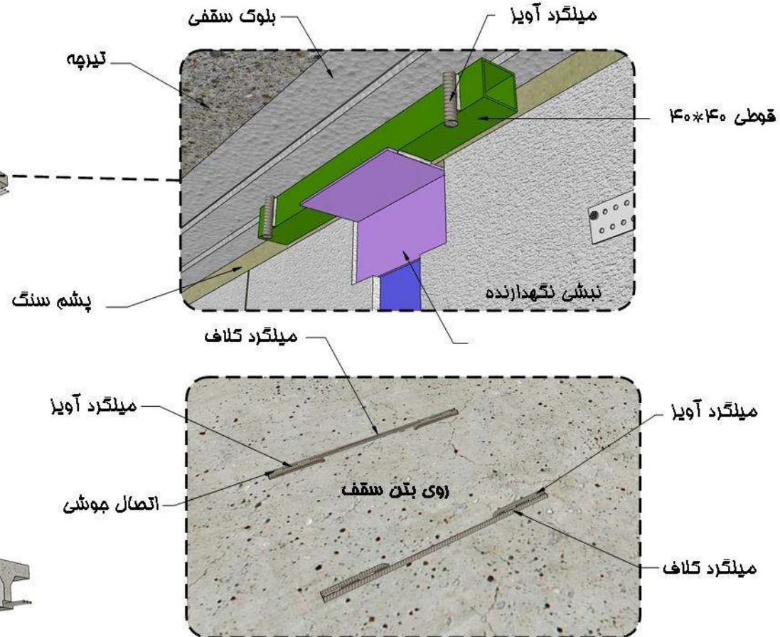
نمونه کلاف کردن میلگرد های آویز به یکدیگر
