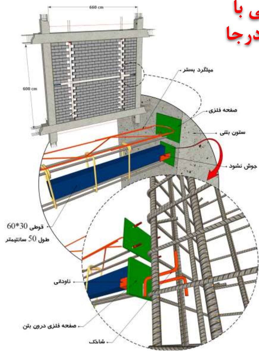
جزئیات اتصال وادر افقی به ستون بتنی
