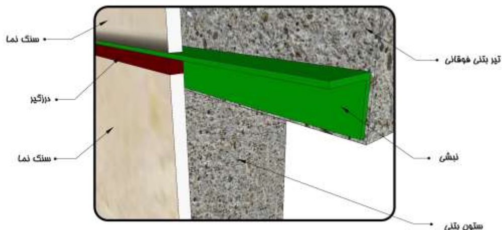
جزئیات اتصال سنگ به نبشی و اجرای درزگیر
