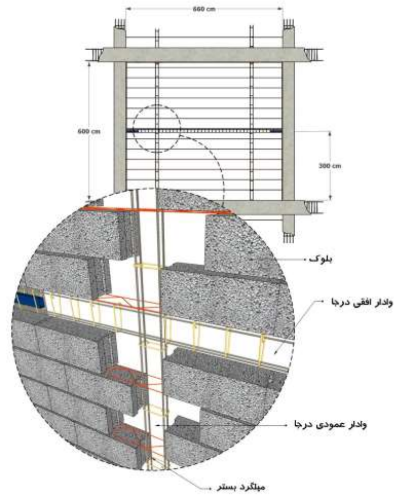
جزئیات اتصال وادر افقی و وادر عمودی
