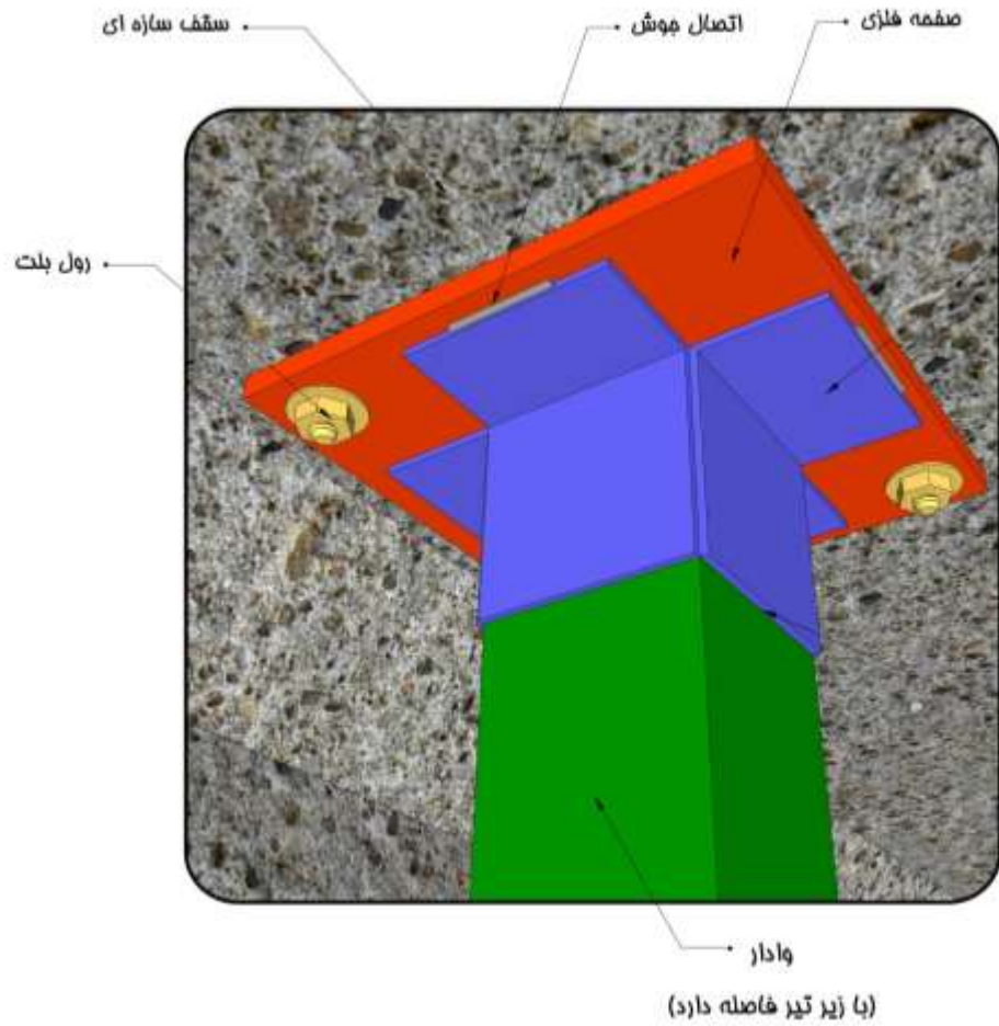
مهار داخل و خارج از صفحه (اتصال تلسکوپی)
