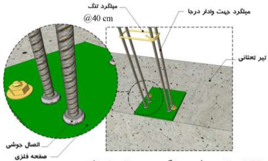
■ اتصال جوشی میلگرد روی تیر تحتانی (پیشنهاد اول)
